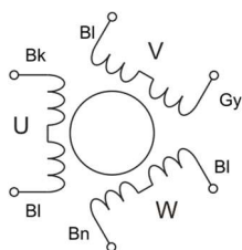
Actual circuit
